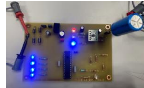
Chargement Cellule Li-Ion (S4 EME)
